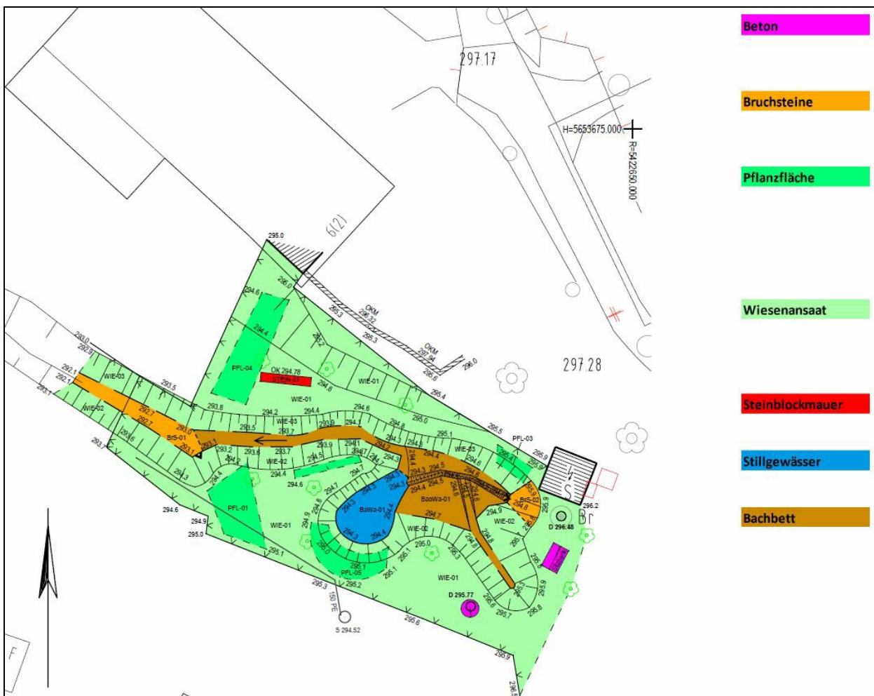
Abb. 3: Schlussvermessung, Lageplan, 11.06.2019
